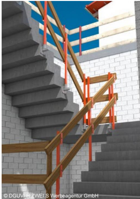
Treppenaufgang mit Seitenschutz
