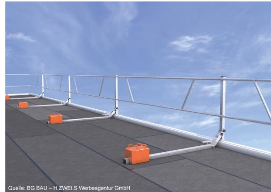
Schutzmaßnahmen gegen Absturz bei Arbeiten an der Dachkante
